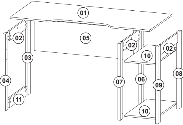
Opção de Montagem Direita Opciones de Armado Derecha Right assembly Option
